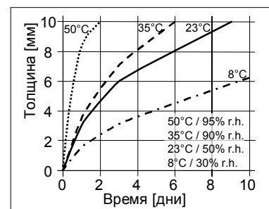
Диаграмма 1: скорость отверждения 1комп. материалов Sikasil®
